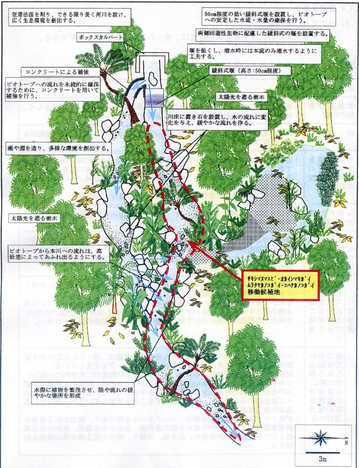
図-7.1.3(5) ビオトープ創出場所における河川水生生物移動候補地イメージ (案)
