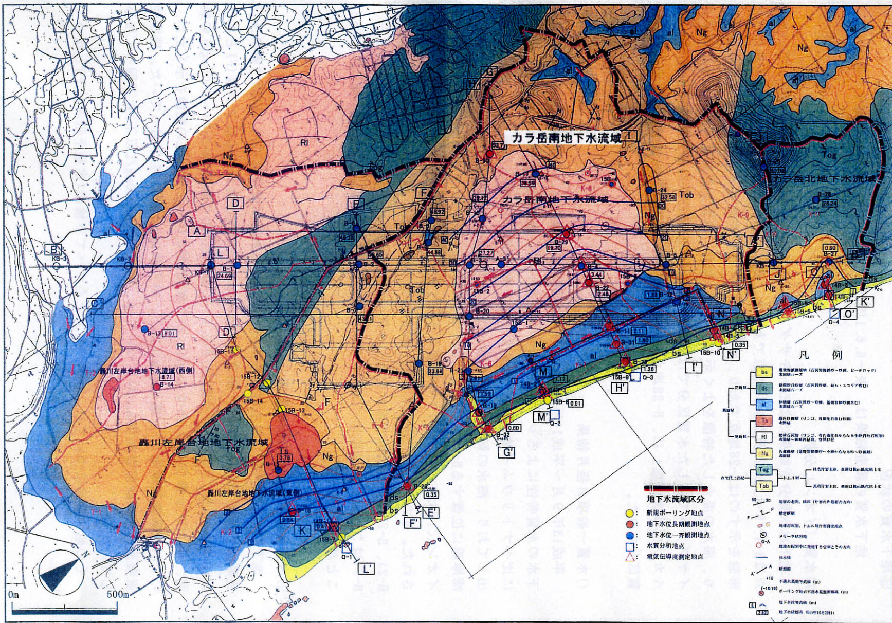
図-6.6.1(1) 地下水調査地点及び水理地質図
