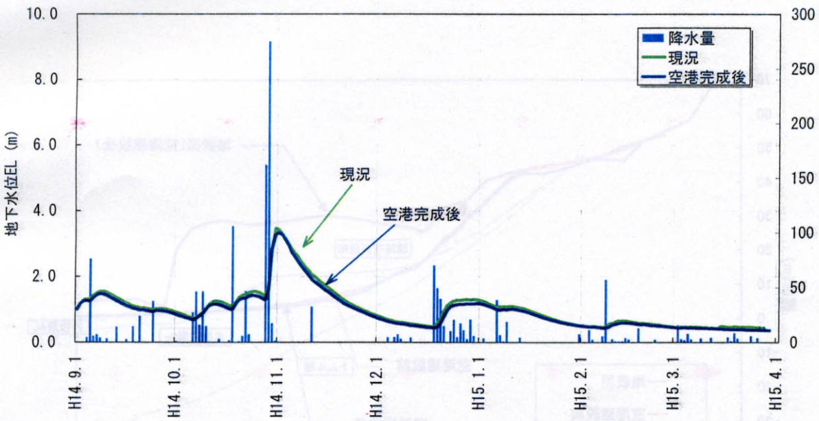
図-6.6.2(11) B-23地点空港建設前と建設後の地下水位変動解析グラフ
