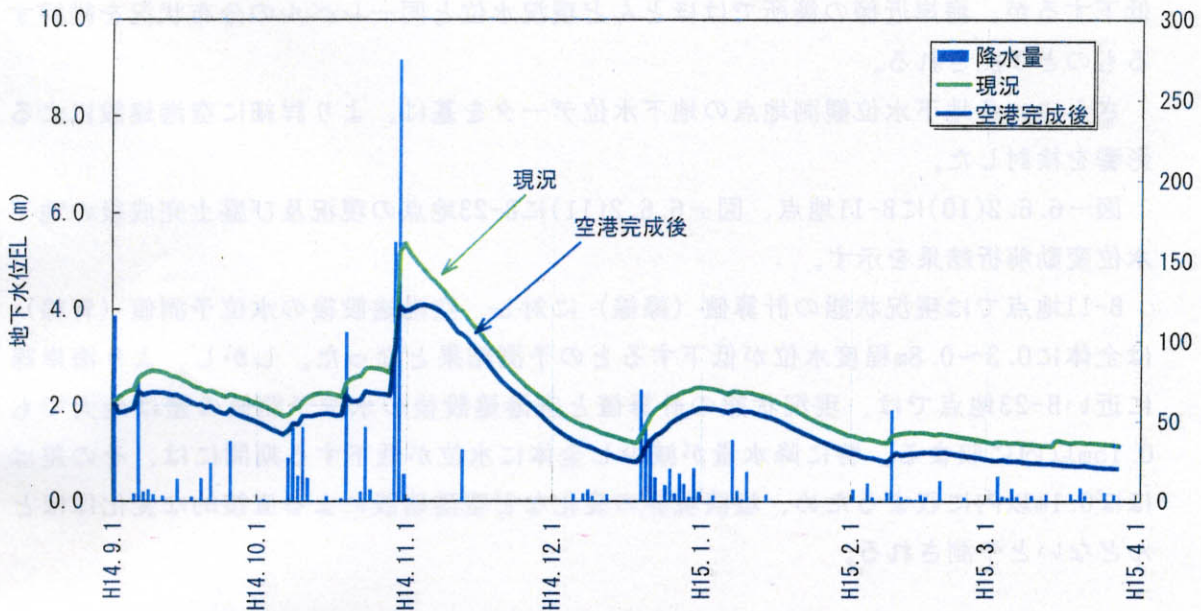
図-6.6.2(10) B-11地点空港建設前と建設後の地下水位変動解析グラフ
