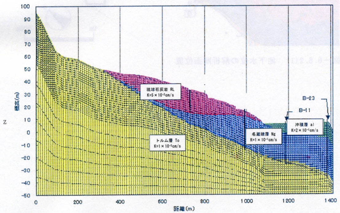
図-6.6.2(3) I-I' 断面モデル要素図
