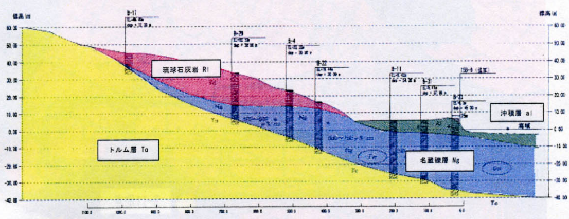
図-6.6.2(2) I-I' 地質断面図
