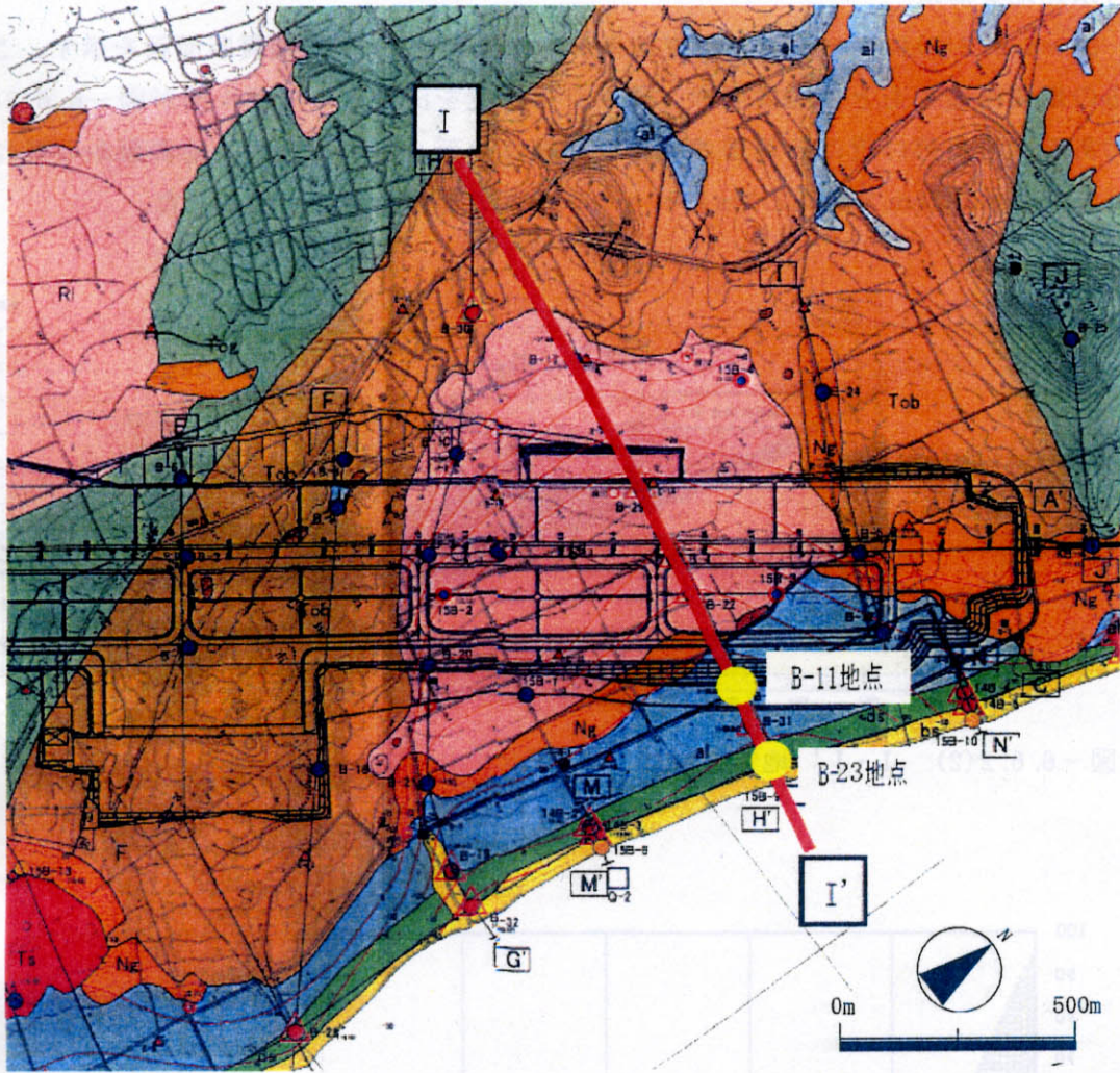
図-6.6.2(1) 地下水位の解析断面位置
