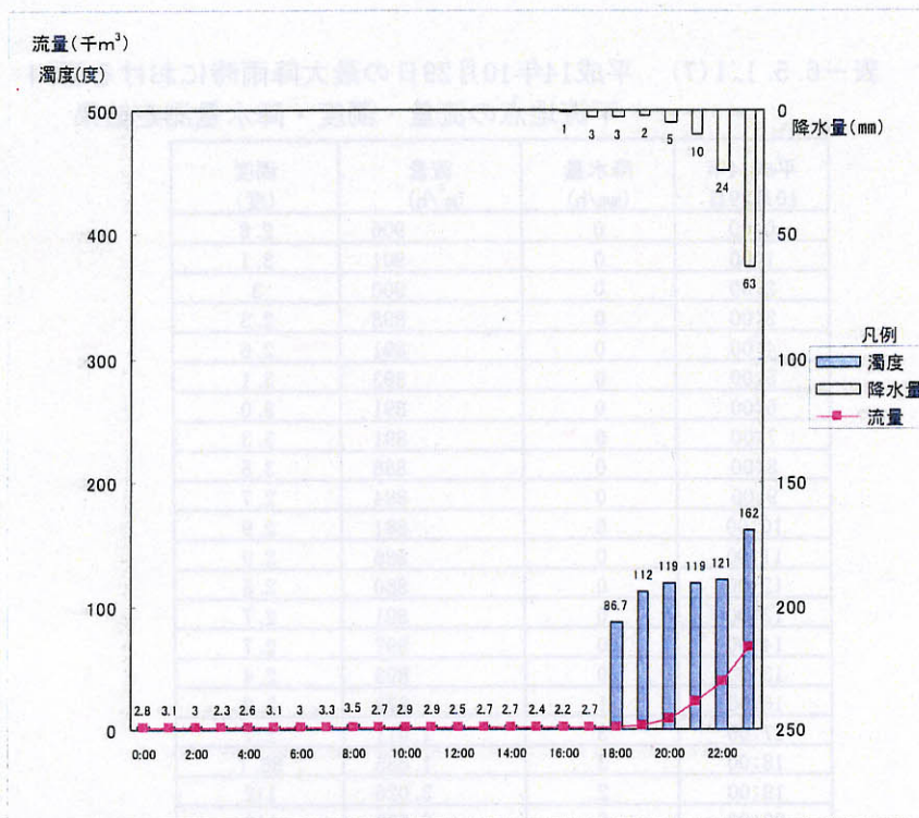
図-6.5.1.1(13) 平成14年10月29日の轟川の流量・濁度・降水量経時変化
