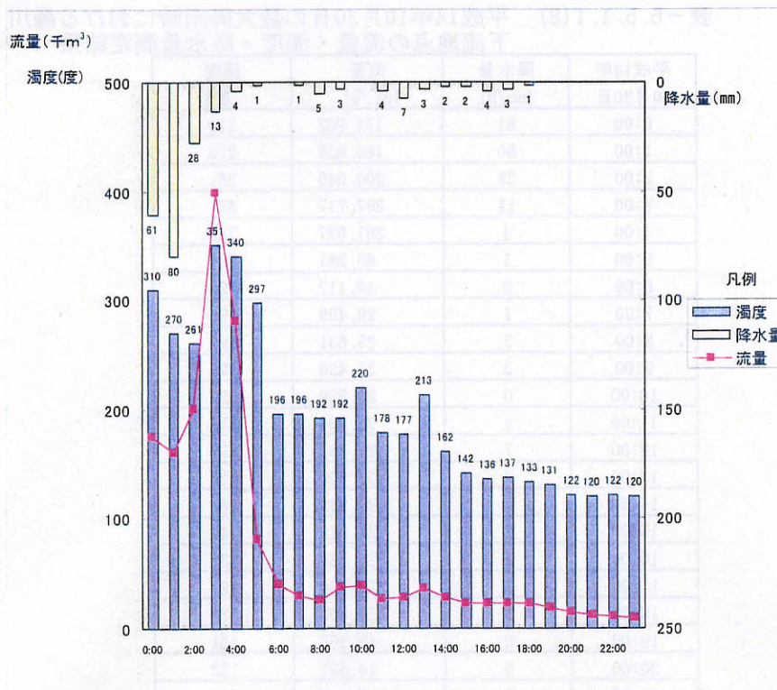
図-6.5.1.1(14) 平成14年10月30日の轟川の流量・濁度・降水量経時変化
