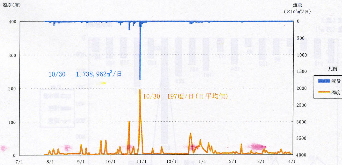
図-6.5.1.1(11) 轟川における日平均濁度と日流量
