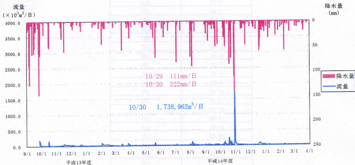
図-6.5.1.1(10) 轟川における日流量と日降水量
