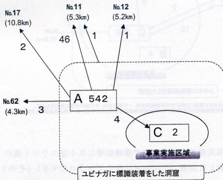
図-6.12.1.2(21) 事業実施区域の5洞窟で標識装着した小型コウモリ類が移動した洞窟 (カグラコウモリ) (その2)
