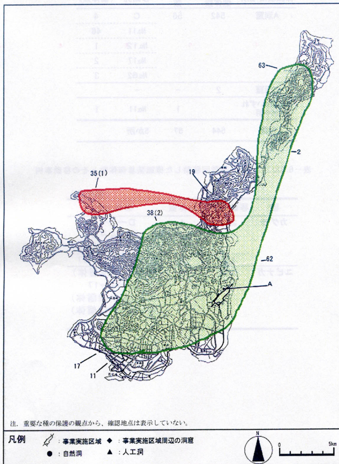
図-6.12.1.1 (59) Neiの遺伝的距離と固定指数 (Fst) に基づきグループ分けした ヤエヤマコキクガシラコウモリのコロニー
