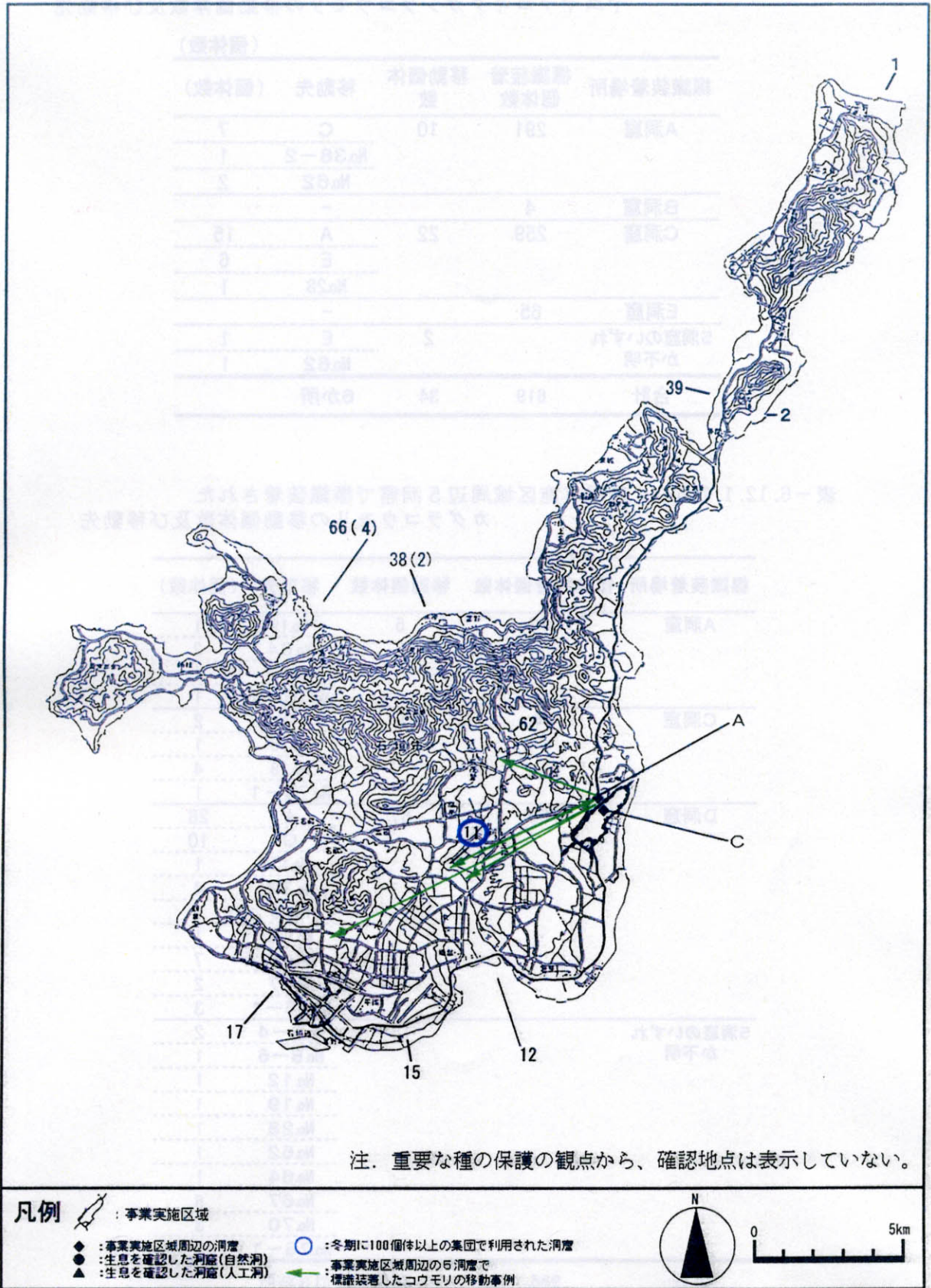
図- 6.12.1.1(58) 石垣島におけるリュウキュウユビナガコウモリの生息状況及び洞窟間の移動事例
