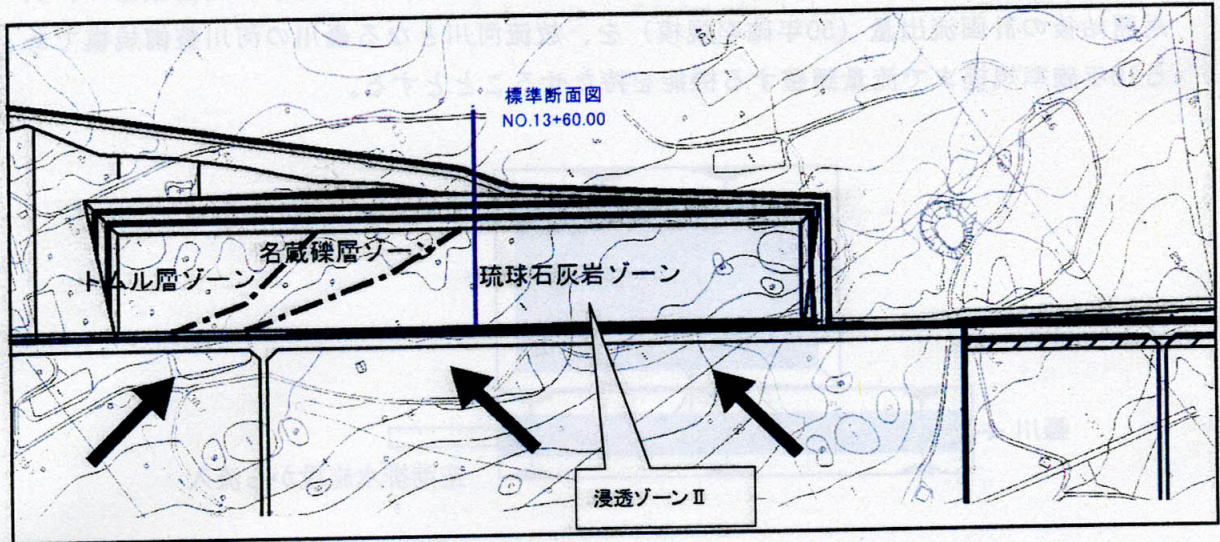
図-6.1.2(6) 浸透ゾーンIIの位置
