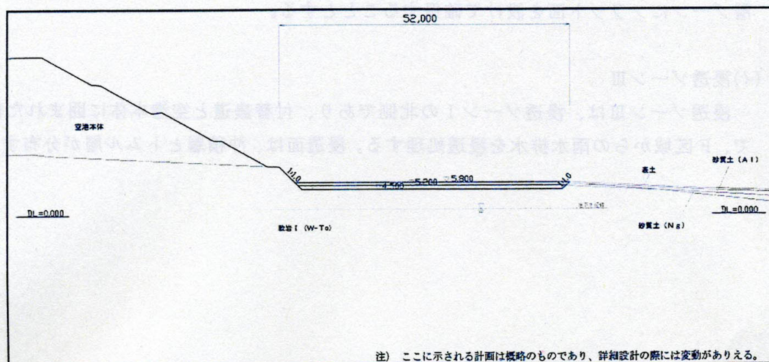
図-6.1.2(5) 浸透ゾーンIIIの標準断面 (NO. 22+0.00、縮尺1:1)
