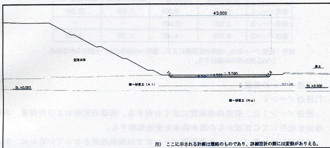
図-6.1.2(4) 浸透ゾーンIの標準断面 (NO. 18+0.00、縮尺1:1)
