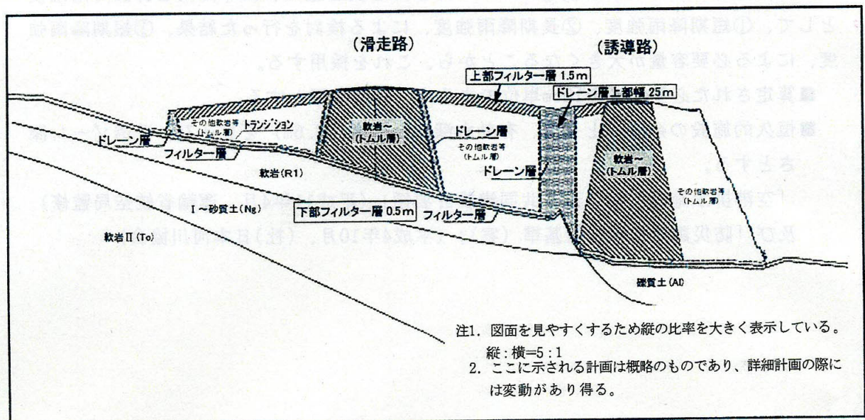
図-6.1.2(1) 盛土構造
