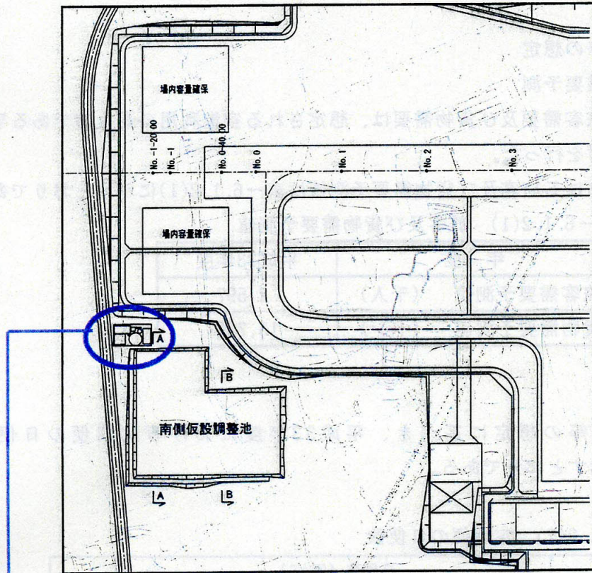
図-6.1.1(10) 南側仮設調整池平面図
