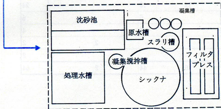
図-6.1.1(11) 機械処理設備の概略設備配置図
