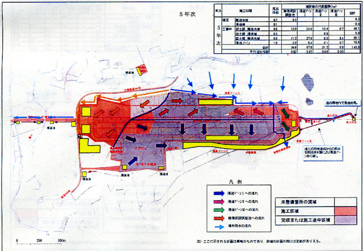
図-6.1.1(6) 年次毎の排水計画 (その2)
