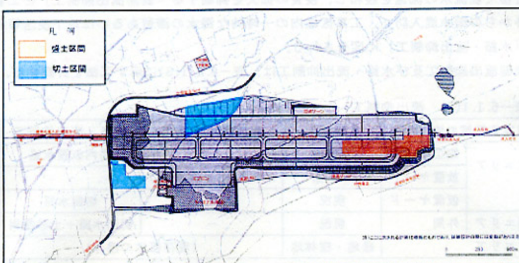
図-6.1.1(5) 年次毎の土工展開 (その2)
