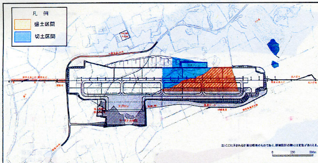
図-6.1.1(5) 年次毎の土工展開 (その1)
