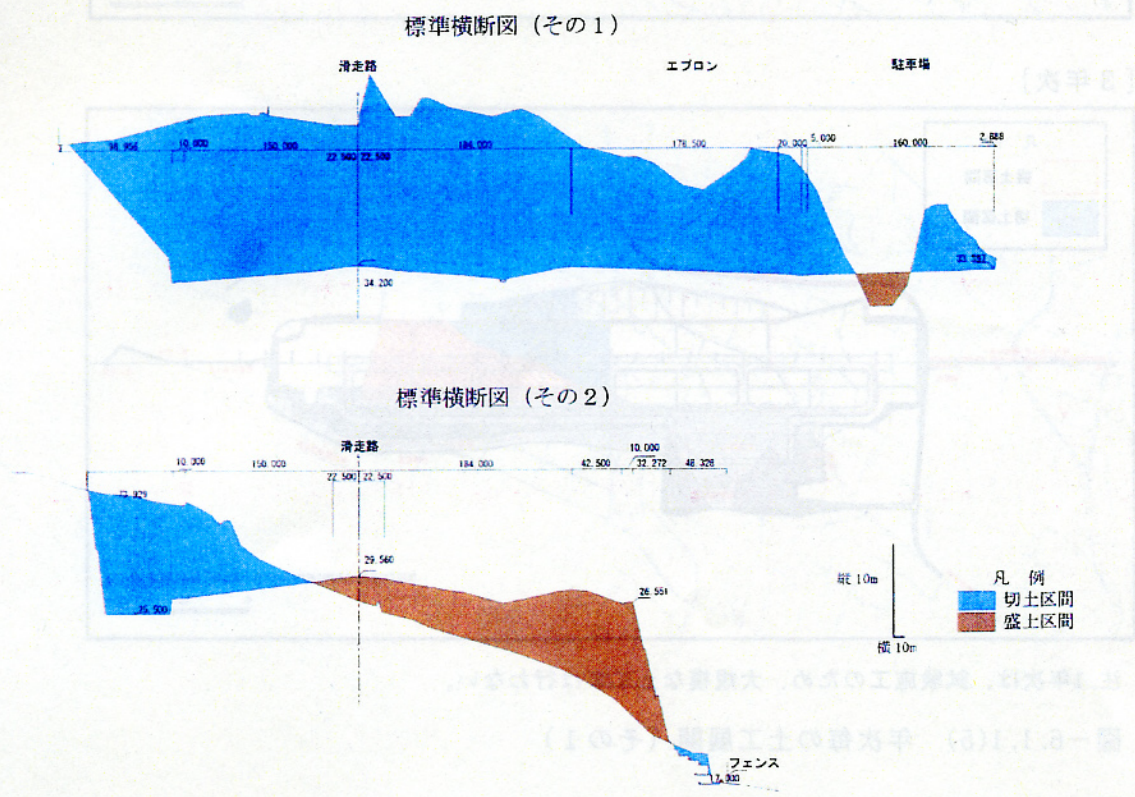
図-6.1.1(3) 縦断面図
