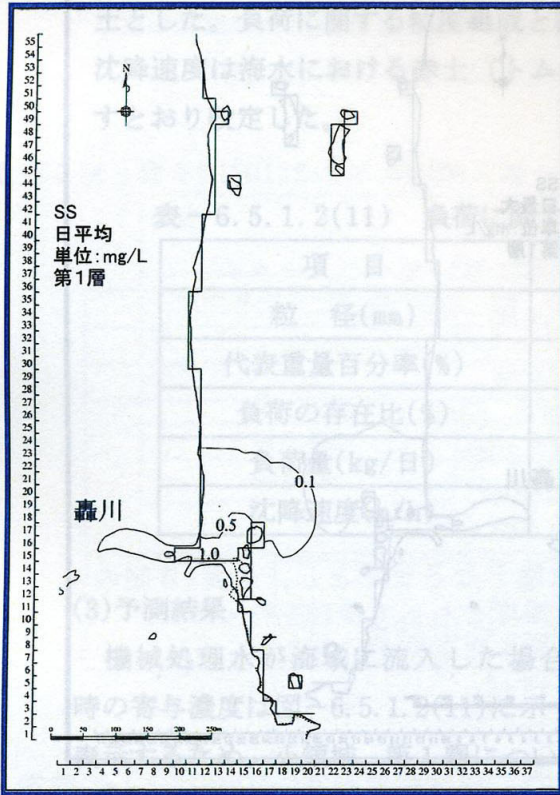
図-6.5.1.2(13) SS濃度分布 (平均潮、平常時、小領域、第1層:平均水面~1.0m層)
