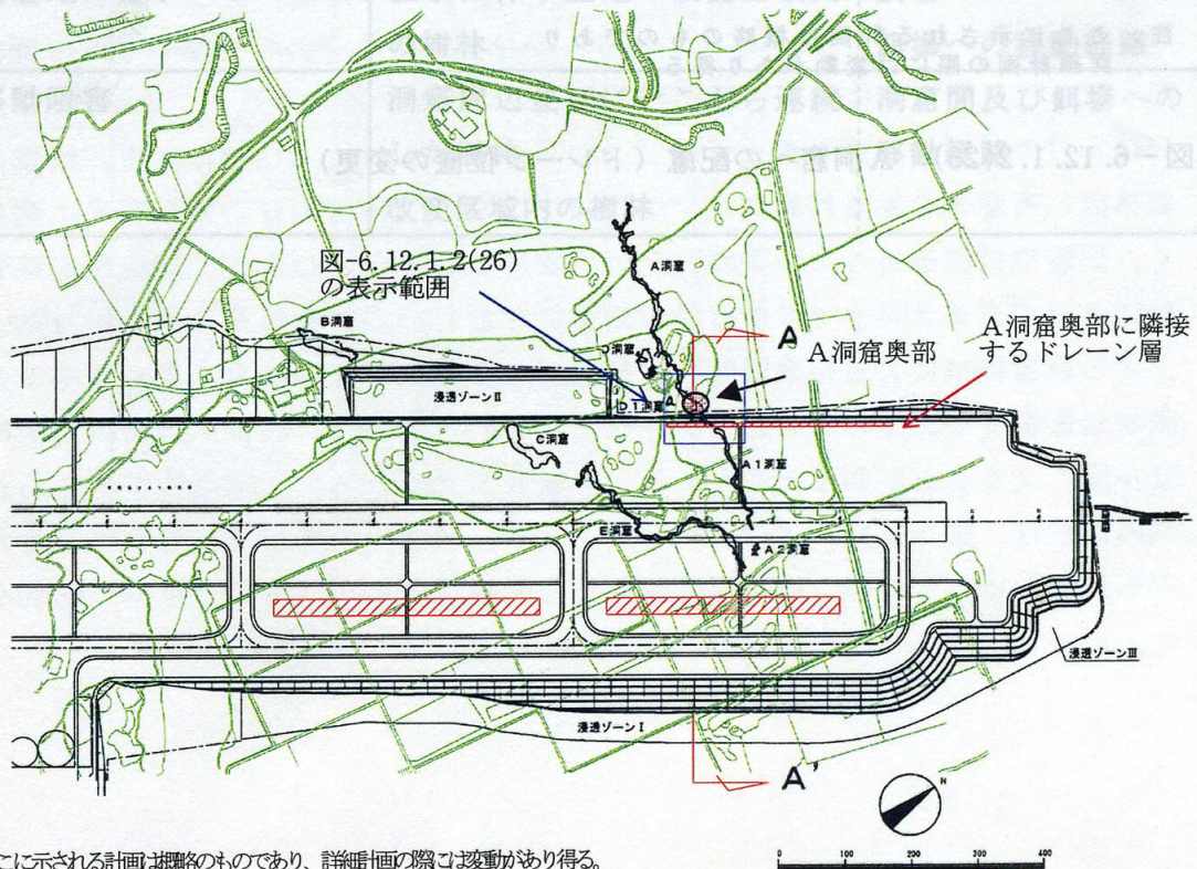
図-6.12.1.2(25) A洞窟と浸透ドレーンの位置関係
