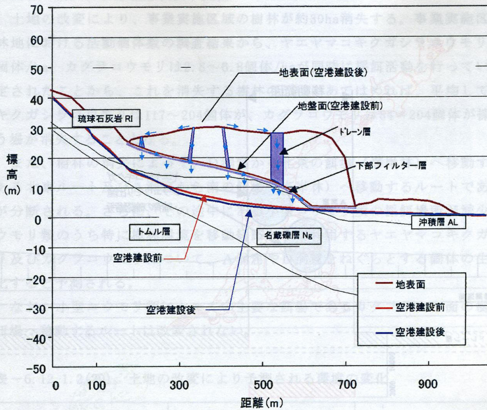
図-6.12.1.2(24) 空港建設前と建設後における10年確率降雨時の地下水分布変化
