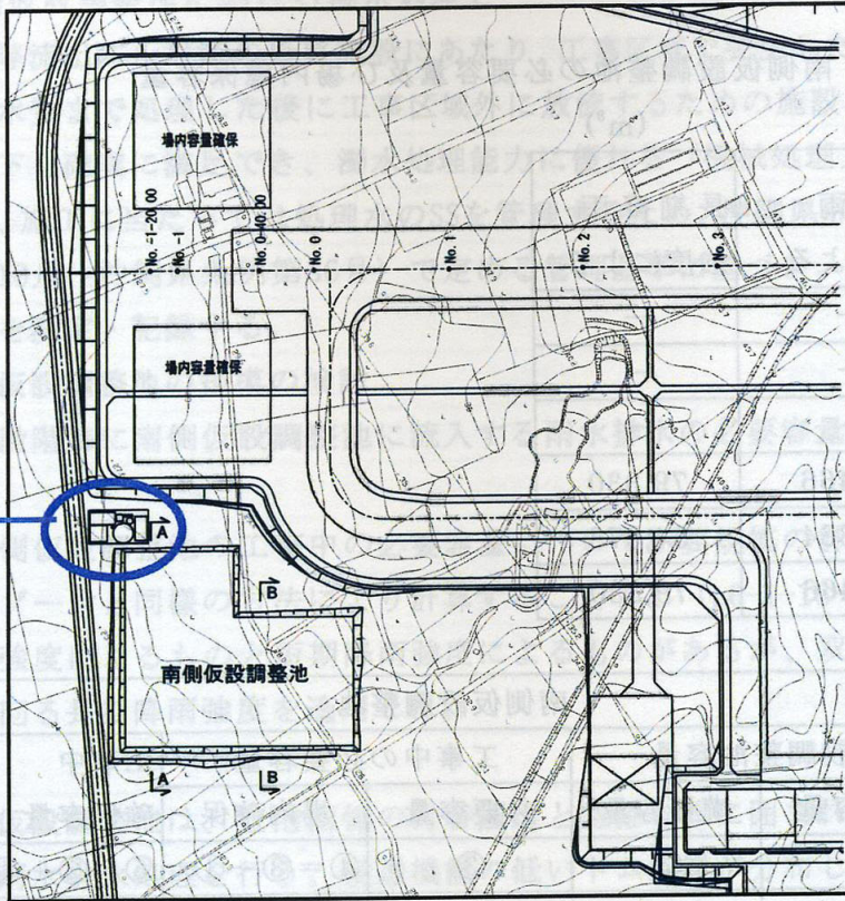
図-6.1.1(23) 南側仮設調整池平面図
