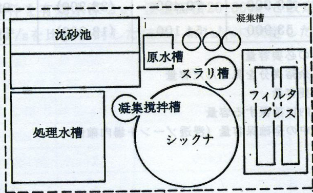
図-6.1.1(24) 機械処理設備の概略設備配置図
