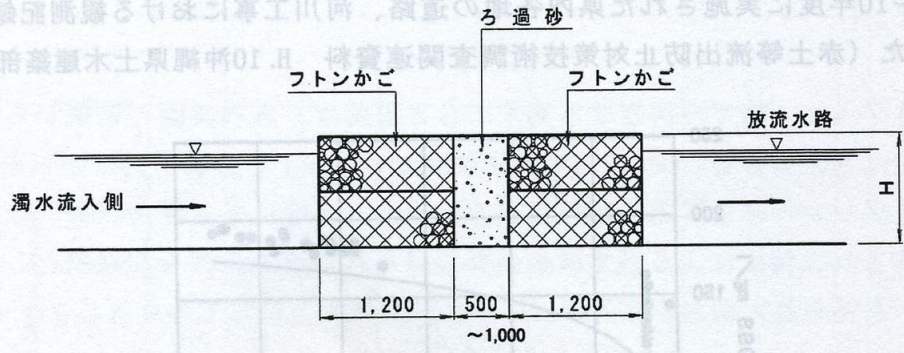
図-6.1.1(20) 受け入れ直前のろ過沈殿処理施設及び砂ろ過堤
